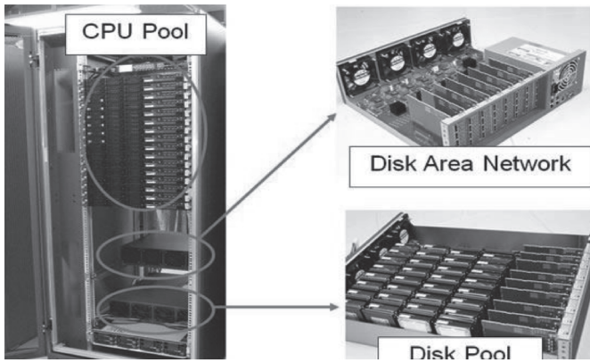
Fig 4: Actual Fujitsu Server Hardware Prototype
